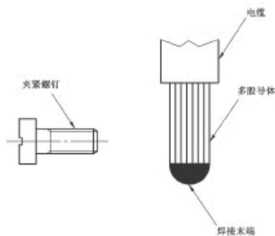
图 28 可以接受的焊接程度的例子
