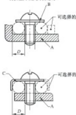
需要垫片或夹片的螺钉
