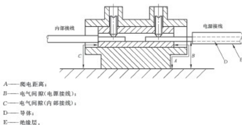
图 24 电源接线端子的爬电距离和电气间隙的图示
