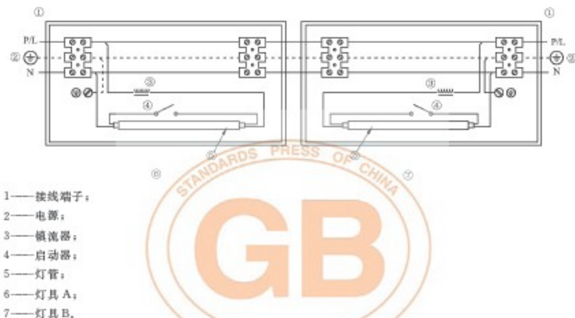
图 20B 术语“通过式布线”在灯具内端接的图例 (灯具被依次连接在 L1、L2、L3 与中线之间时,可用三相通过式布线)
