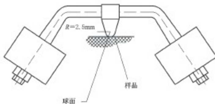
图 10 球压装置
