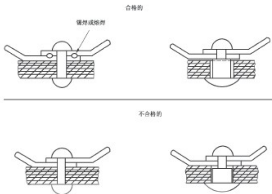
图 17 电气连接件结构图
