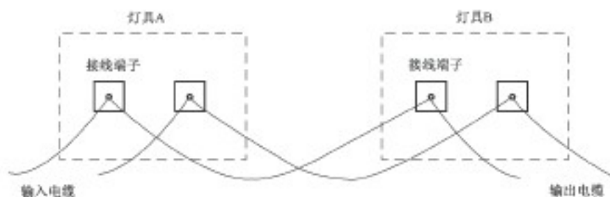
图 20A 术语“环路安装”(转接供电)的图例
