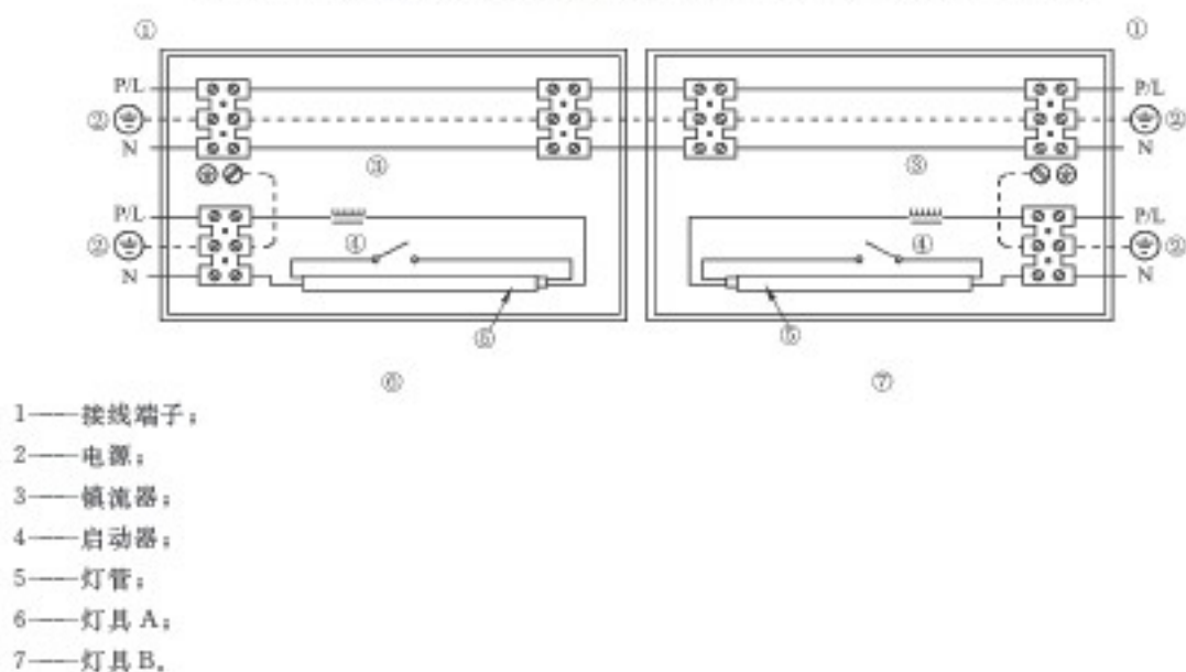
图 20C 术语“通过式布线”不在灯具内端接的图例
