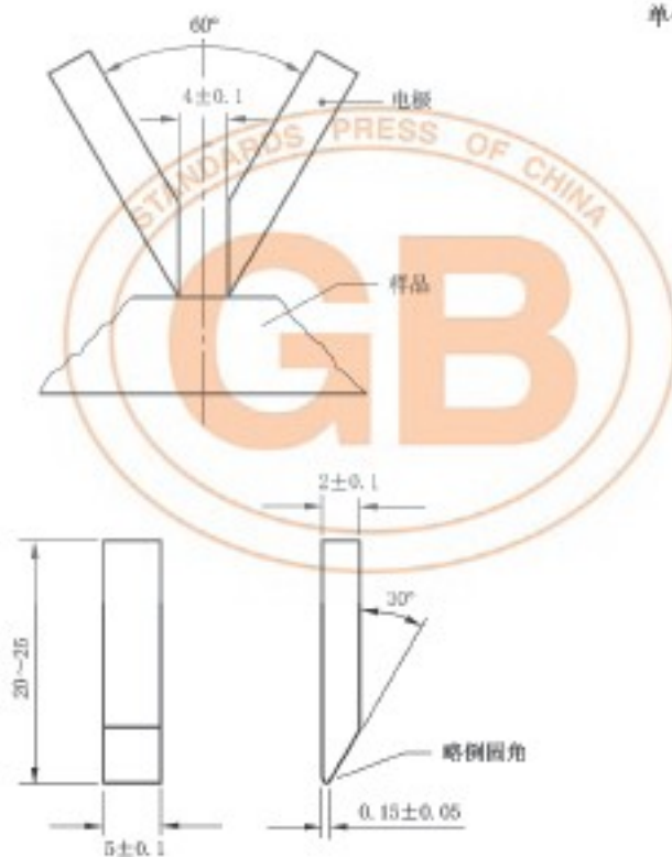
图 11 耐起痕试验用电极的尺寸和安装布局
