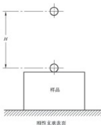
图 21 球冲击试验的装置
