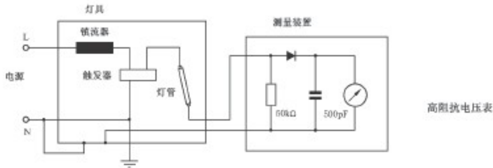
图 26 插入期间安全的测试电路
