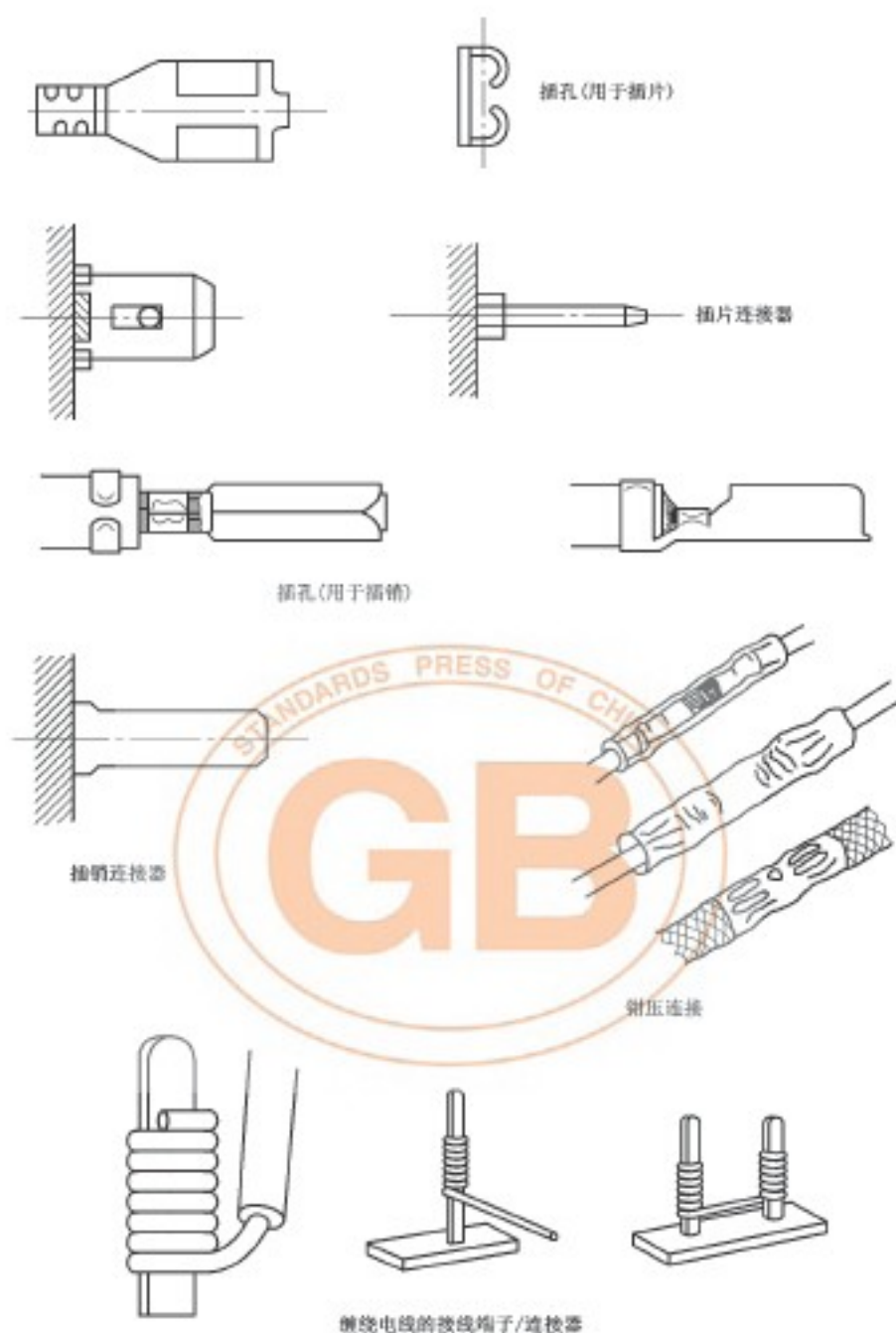
图 19 无螺纹接线端子的其他例子
