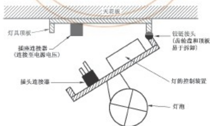
图 31 插头/插座连接的电气—机械接触系统
