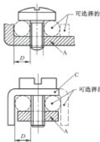
不需垫片或夹片的螺钉
