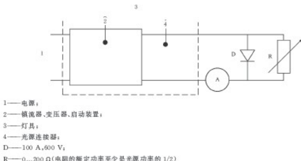
图 C.3 某些高压钠灯和某些金属卤化物灯整流效应的试验线路
