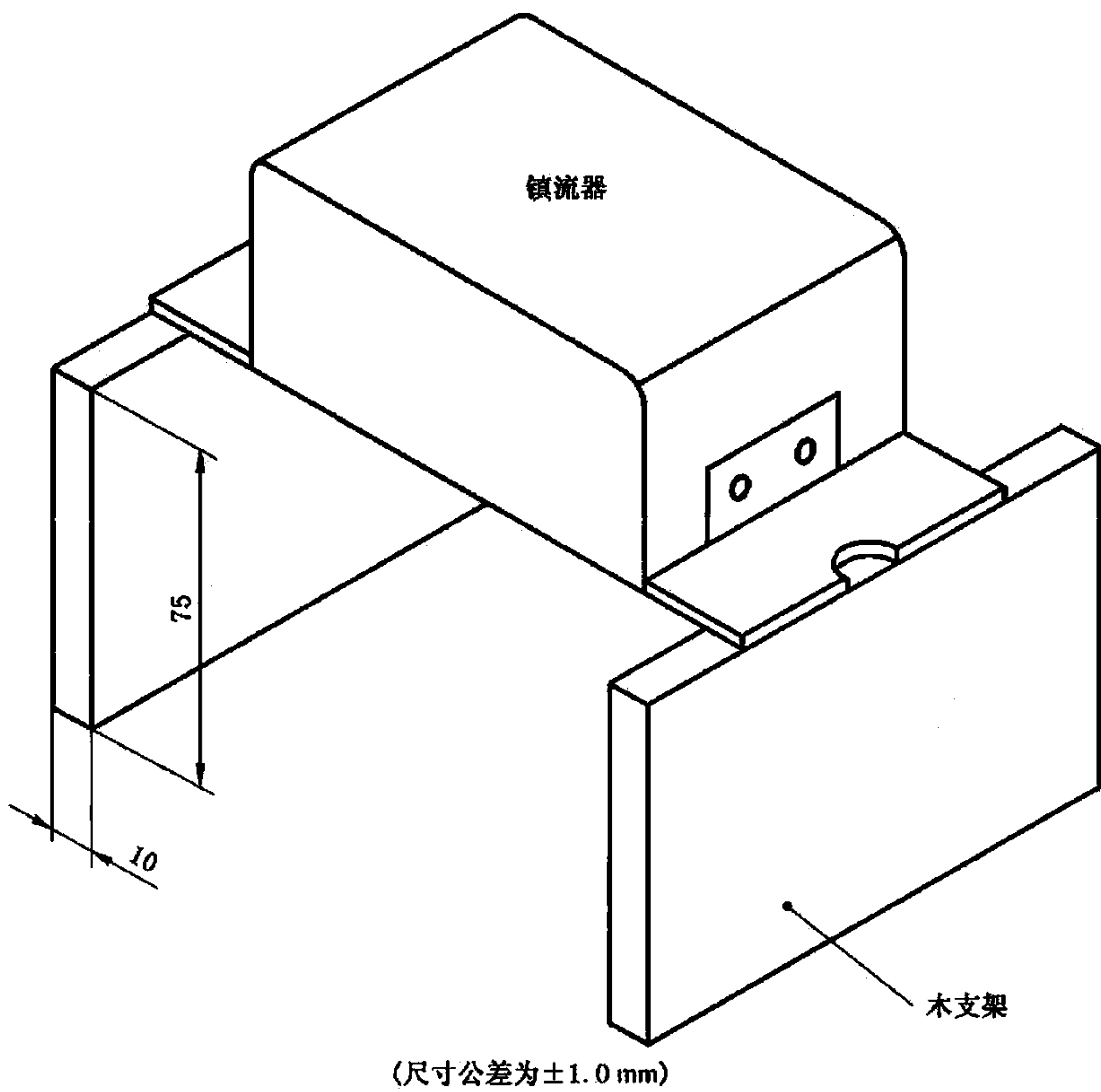
图 H.1 加热试验样品配置图
