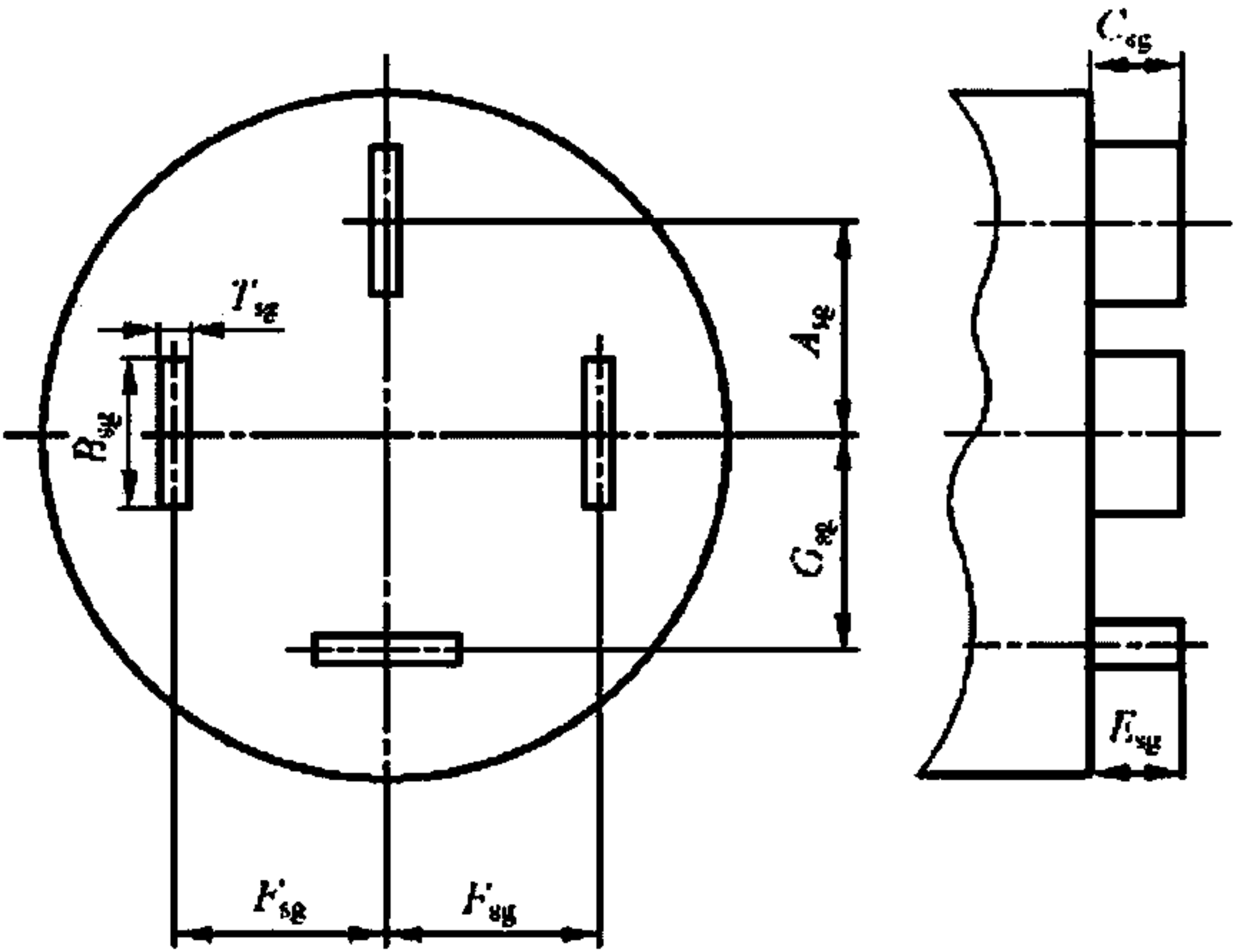
图 7 三相插座止规
