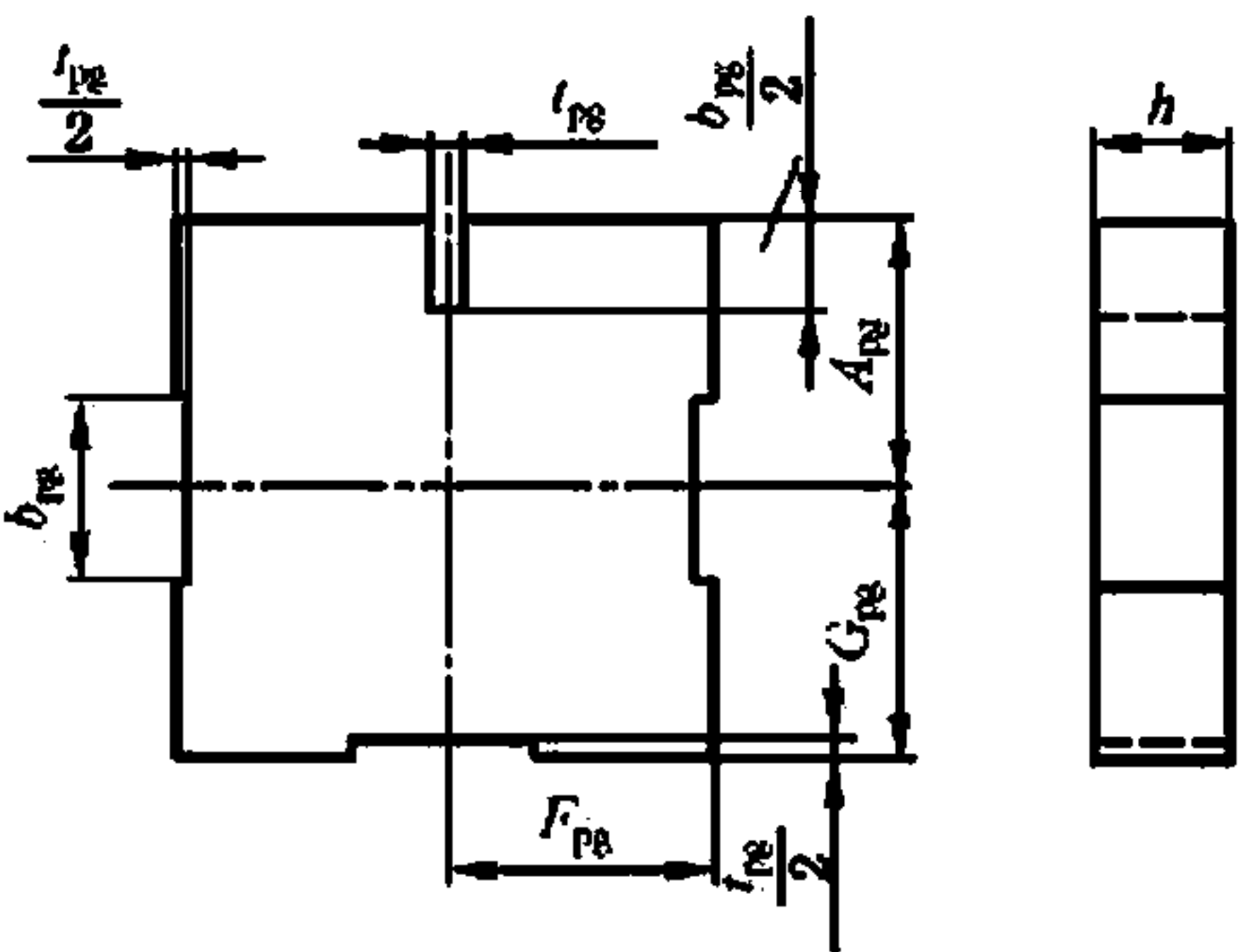
图 3 三相插头内量规
