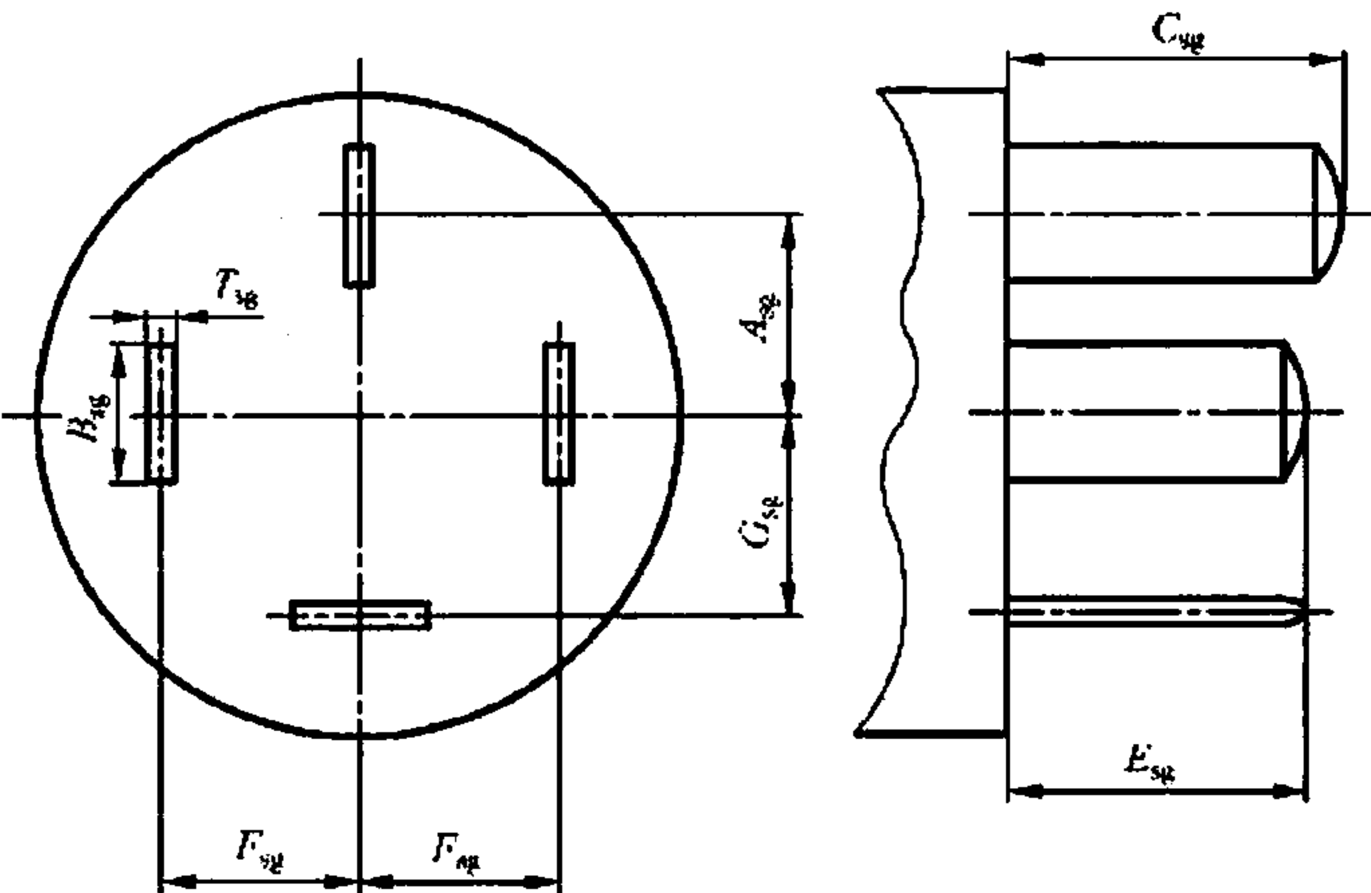
图 6 三相插座最小通规 表 6 三相插座最小通规尺寸
