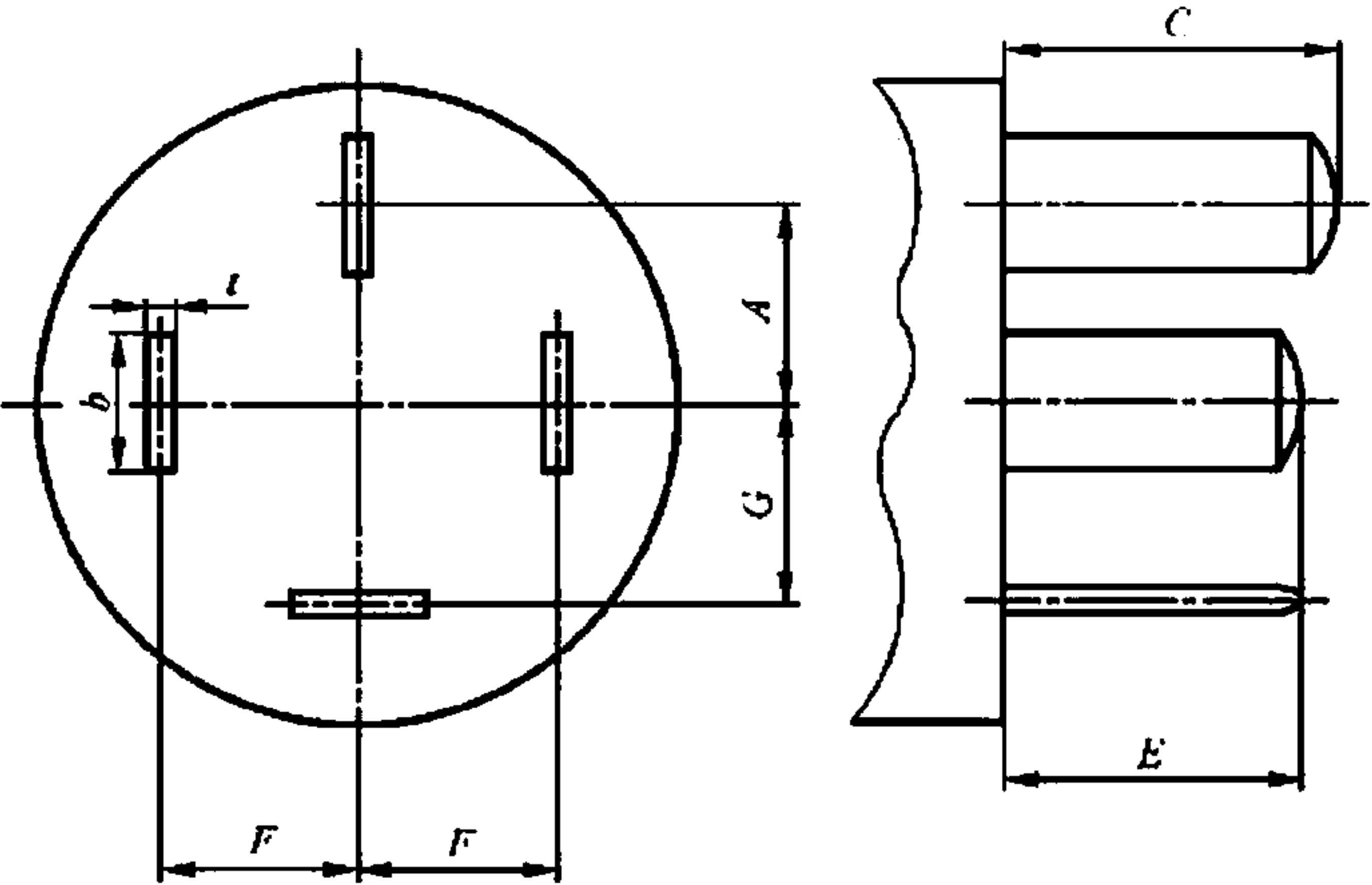
图 1 三相插头
